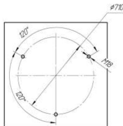
Схема расположения фундаментных болтов
